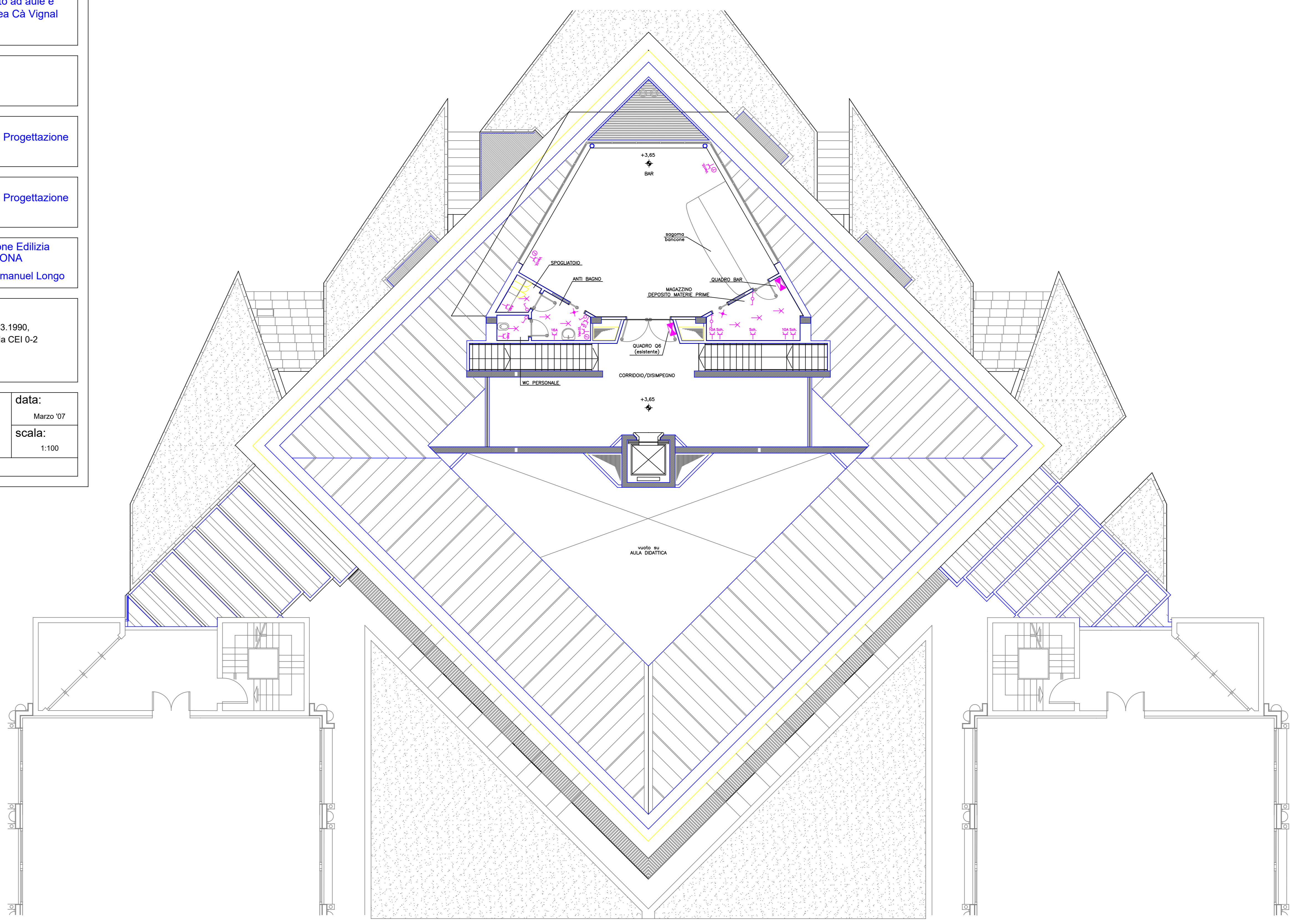
PIANO PRIMO SCALA 1:100
